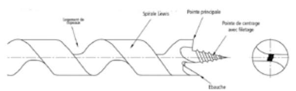
Mèches à bois à simple spirale Lewis
