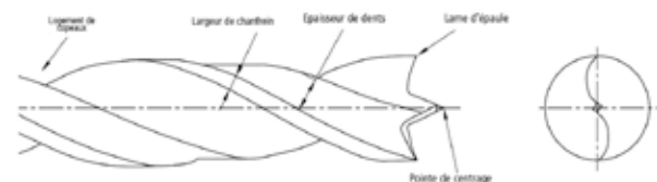
Mèches à bois
